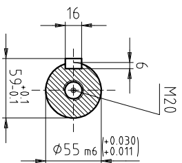
SEZ. A-A
