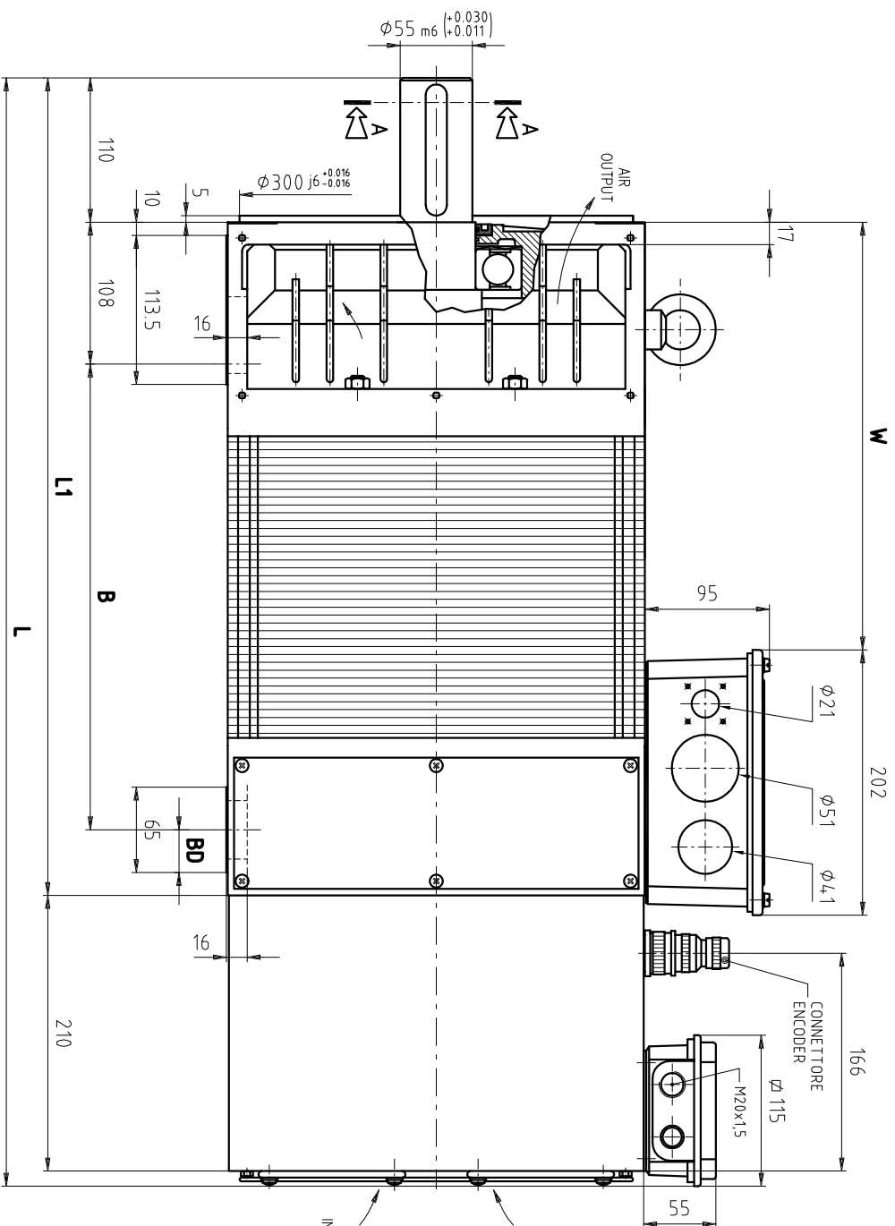
SEZ. A-A
